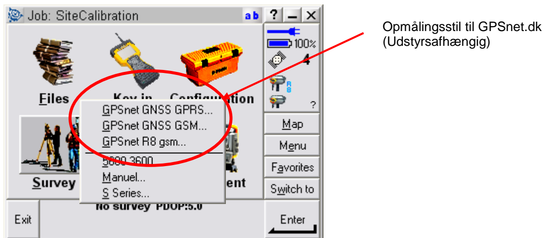
Figur 2 Opmåling, her kan vælges den måde (opmålings-stil) du vil "ringe" GPSnet.dk op på.
